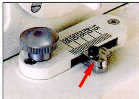
缝制长度的调整装置
