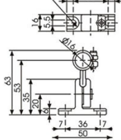
Bracket D-type / 燈座
