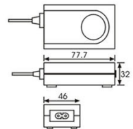
Adapter < LA-05A > / 變壓器
